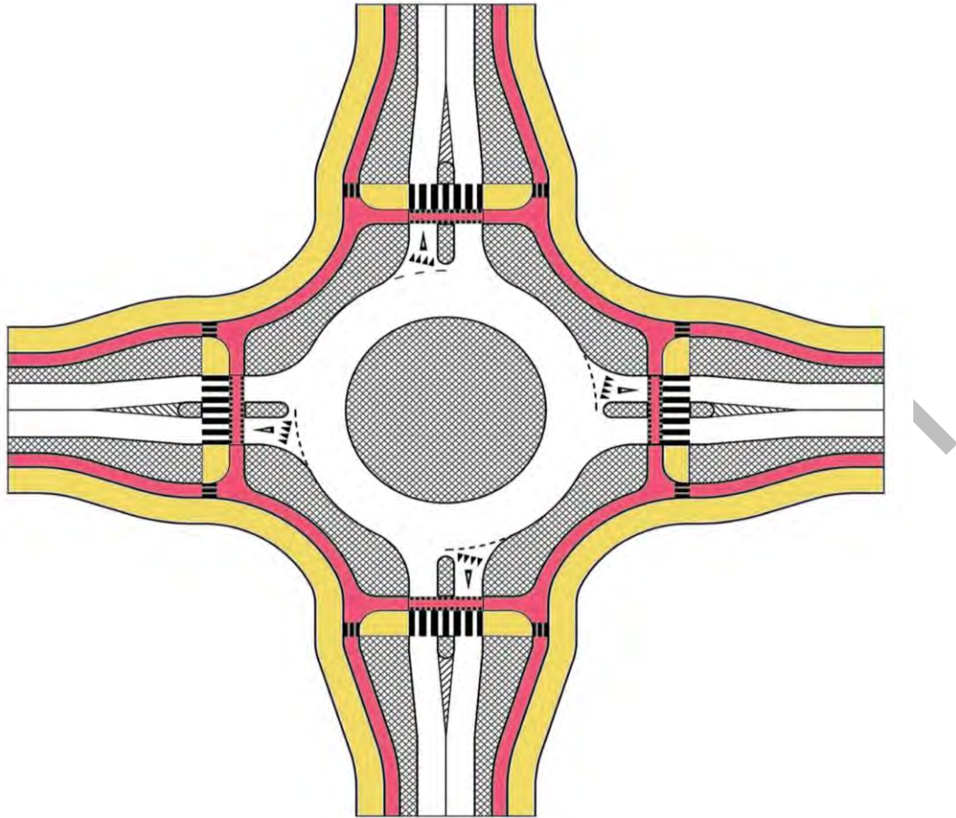
35-р зураг – Зорчих хэсгээс тусгаарлагдсан унадаг дугуйн зам
