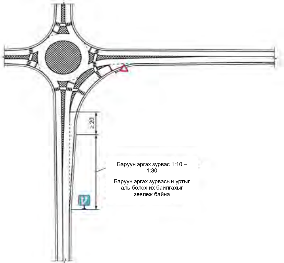
20-р зураг - Хөдөлгөөнийг залж баруун эргэх зурвас
