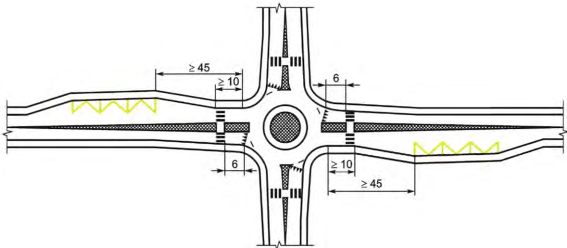
31-р зураг — Тойрог уулзвараас гарах хэсэг дээрх автобусны буудлыг төлөвлөх зай
