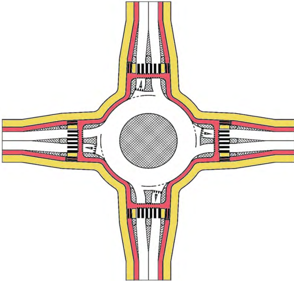
34-р зураг – Тойргийн зорчих хэсгээс нарийн тусгаарлагч дээр байрлуулсан дохионы шонгоор тусгаарласан дугуйн зурвас
