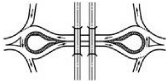
г) Бүрэн бус хэлбэрийн давхар зам дээрх тойрог уулзвар
