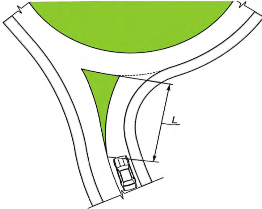
15-р зураг – Чиглүүлэгч арлын уртыг тодорхойлох схем
