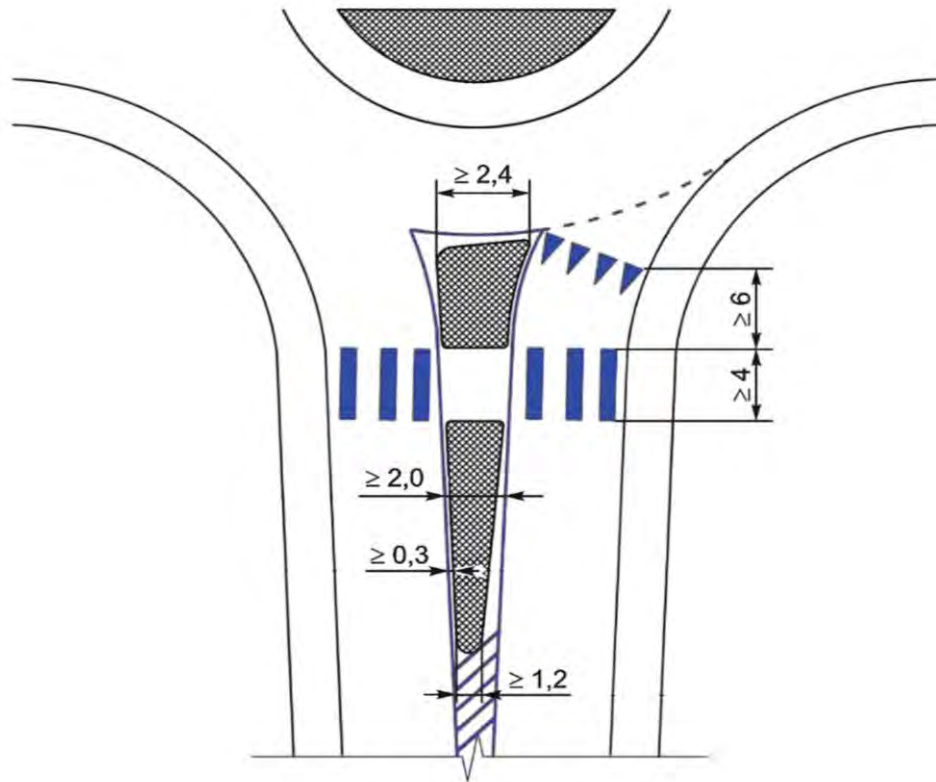
16-р зураг - Чиглүүлэгч арал төсөллөх жишээ
