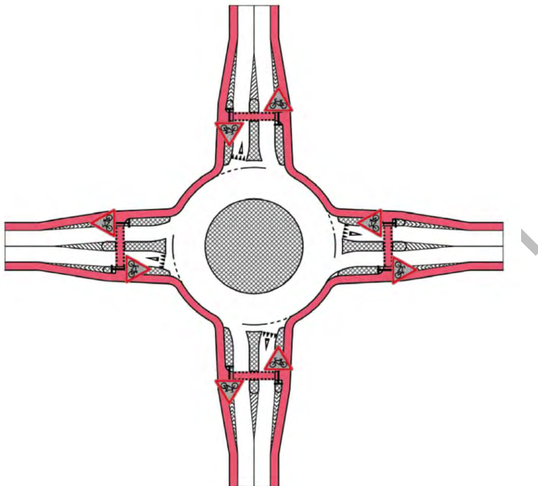
32-р зураг — Тойргийн зорчих хэсэг дээрх унадаг дугуйн зурвас
