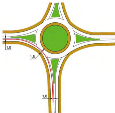
в) Баруун гар тийш эргэх хөдөлгөөн
