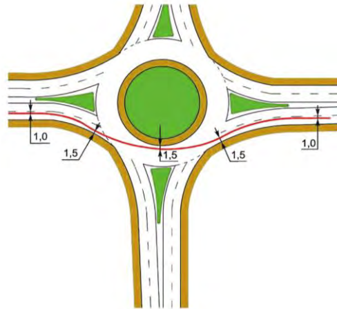
б) Хоёр зурвастай тойрог уулзварыг шулуун чиглэлээр нэвтрэх
