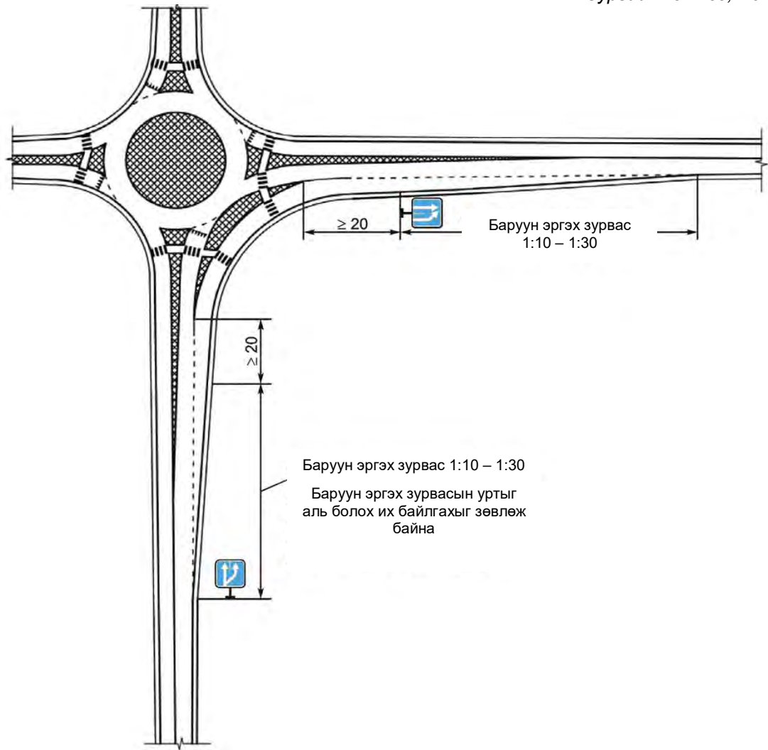
19-р зураг - Нэмэлт зурвасын тусламжтайгаар баруун эргэн зурвас
