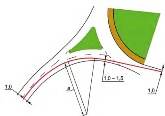
г) - Ойртох хэсэг дээрх чөлөөт явалтын хамгийн бага радиусыг (R1) тодорхойлох
