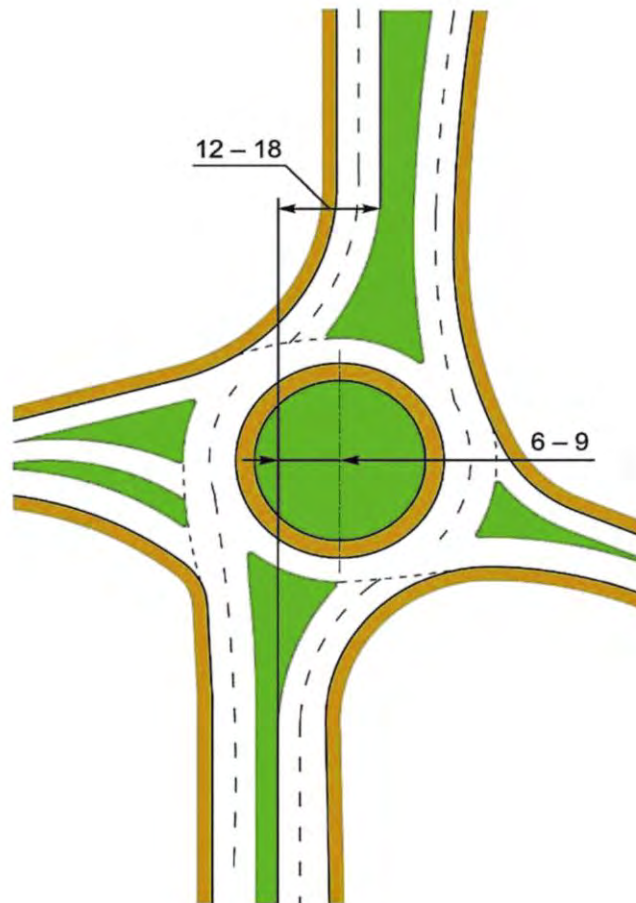
14-р зураг - Орох радиусыг багасгахын тулд ойртох тэнхлэгийг тойрог уулзварын төвөөс зүүн тийш шилжүүлэх жишээ
