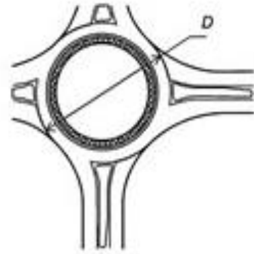
б) дунд зэргийн диаметртэй тойрог уулзвар ( D = 30 - 50 м)
