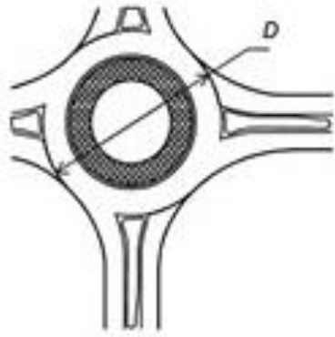
а) бага диаметртэй тойрог уулзвар ( D=24 м - 30 м)
