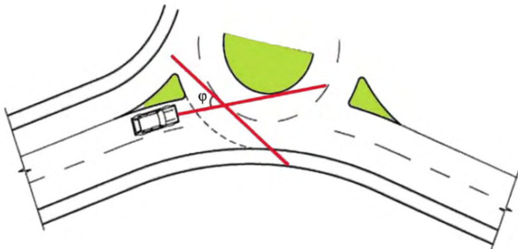
10-р зураг - Тойрог уулзвар руу оролтын бага өнцөг (<20°)
