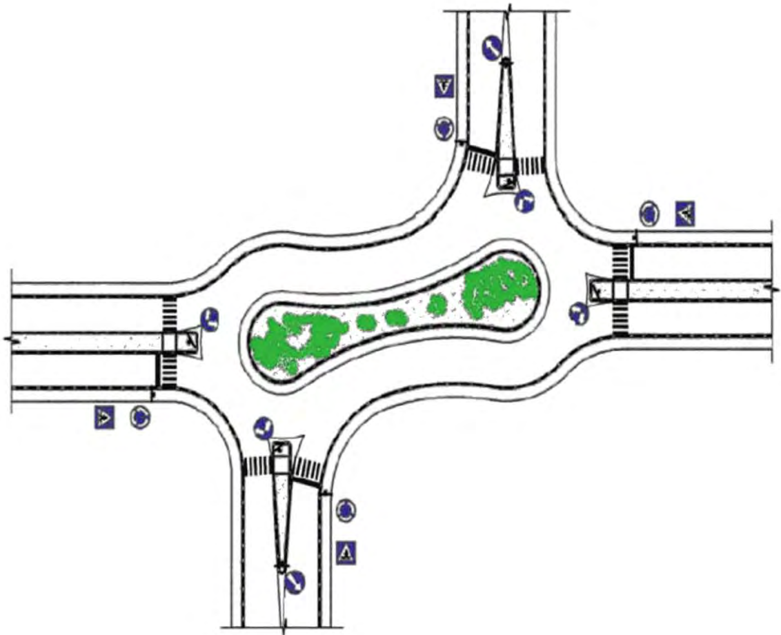
3-р зураг - Сунасан төв арлын тусламжтайгаар шатласан 8-ын тоо хэлбэрийн тойрог уулзварын төлөвлөлтийн шийдэл
