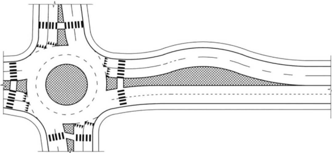
17-р зураг - Тойрог уулзвар руу ойртох хэсэг дээрх хурдыг багасгах шаардлагатай үед урвуу дугуй муруйнуудын тусламжтайгаар тэдгээрийн хооронд шулуун оруулга хийлгүй чиглүүлэгч арлыг төсөллөх жишээ
