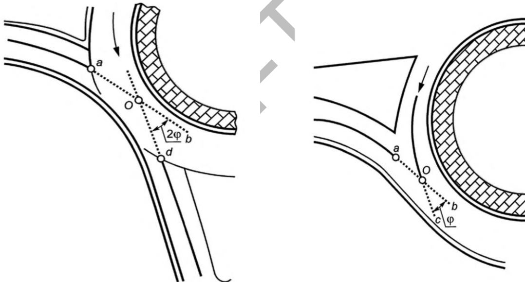
а) Нийлэх чиглэлүүдийн хоорондох зай 30м-ээс бага байх үеийн орох өнцөг
