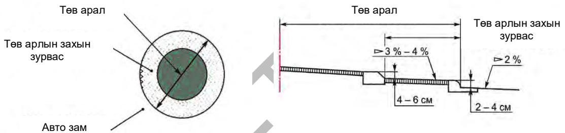
а) Хязгаарын зурвастай төв арлын план
